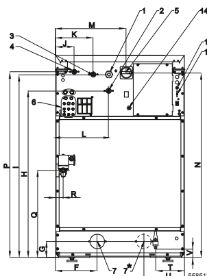
RÜCKANSICHT
