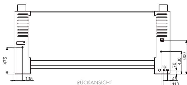
RÜCKANSICHT
